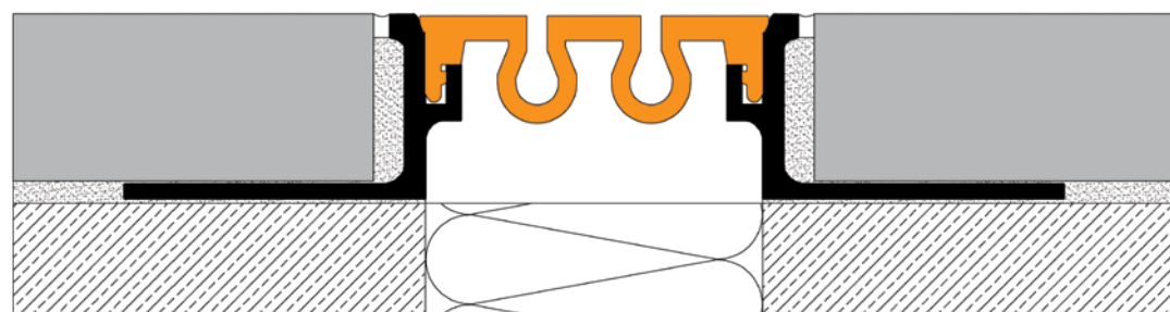
11. ábra – Előregyártott szerkezeti dilatációs profil vázlata
