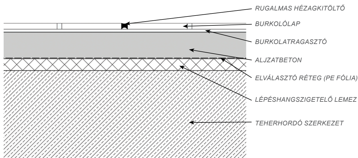
9. ábra – Burkolatdilatáció vázlata
