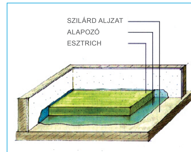
kötött esztrich
