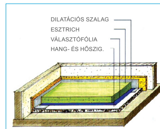
úsztatott esztrich
