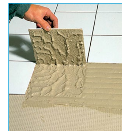
Burkolás folyékonyágyas ragasztóba
